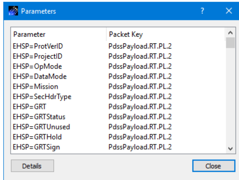
Figure 37 Parameters Dialog
